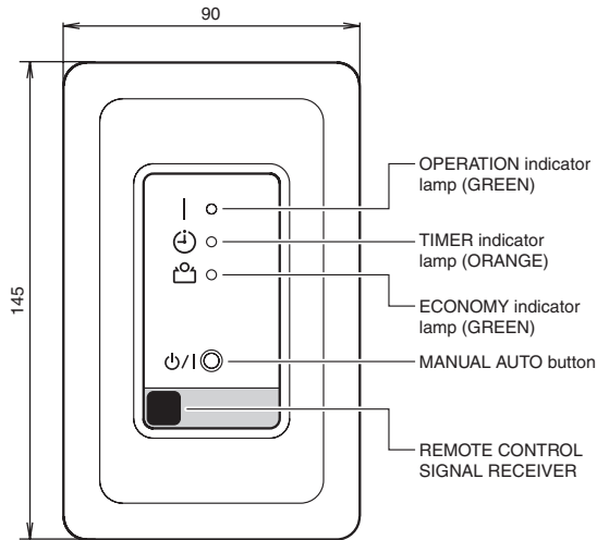
Dimensions
